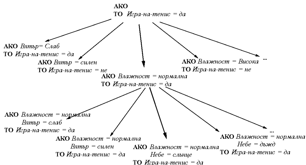
Фиг. 5-1. Дървото на търсене
