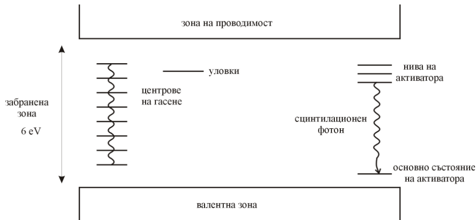
Фиг. ПЗ. Схема на електронните нива в неорганичен кристал с активатор.
