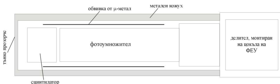
Фиг. П1. Схема на сцинтилационен детектор
