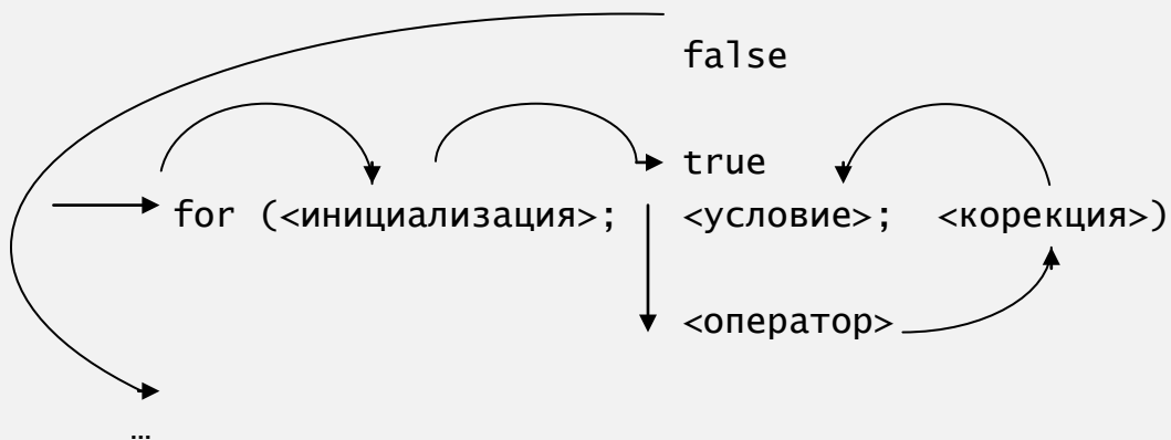
фиг. 4.9 Оператор за цикъл for
