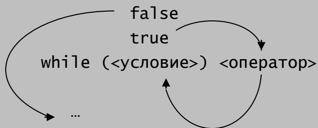
фиг. 4.10 Оператор while
