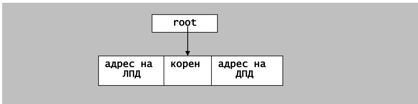
Фиг. 16.1 Свързано представяне на двоично дърво
