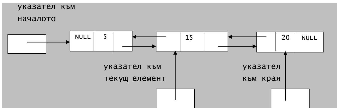
Фиг. 15. 5 Представяне на свързан списък с две връзки
