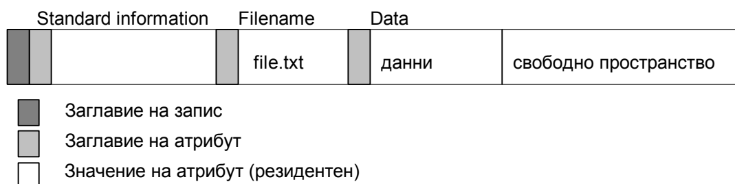
Фиг.20. MFT запис за файл само с резидентни атрибути
