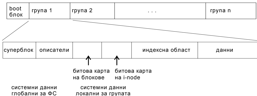
Фиг.13. Разпределение на дисковото пространство в ext2/ext3 на LINUX
